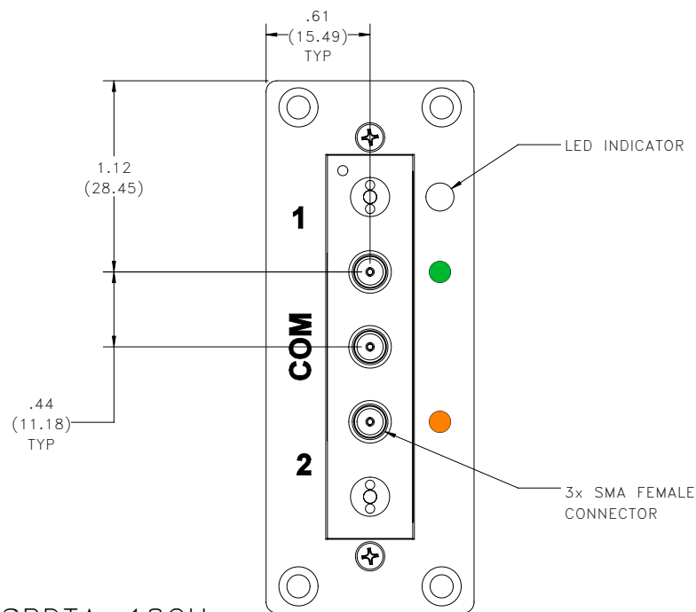
SPDTA-18GHz
