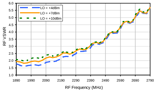
RF VSWR
