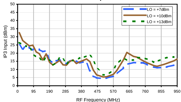
IP3 Input
