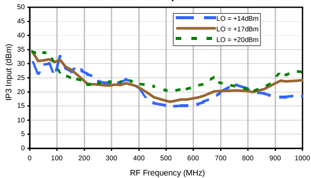
IP3 Input
