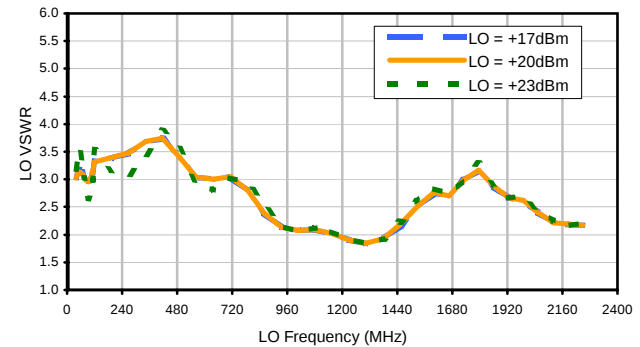
LO VSWR
