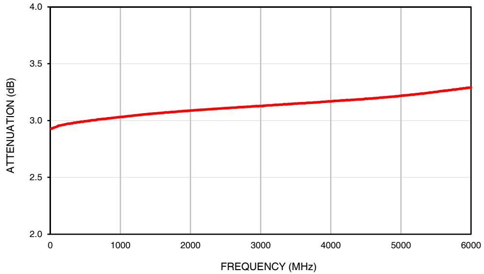
ATTENUATION
