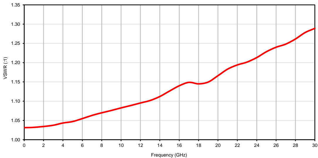
VSWR
