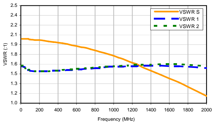
VSWR
