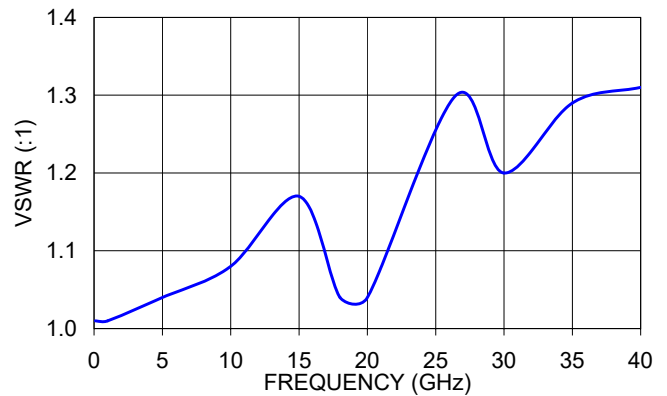
BW-K20-2W44+ VSWR
