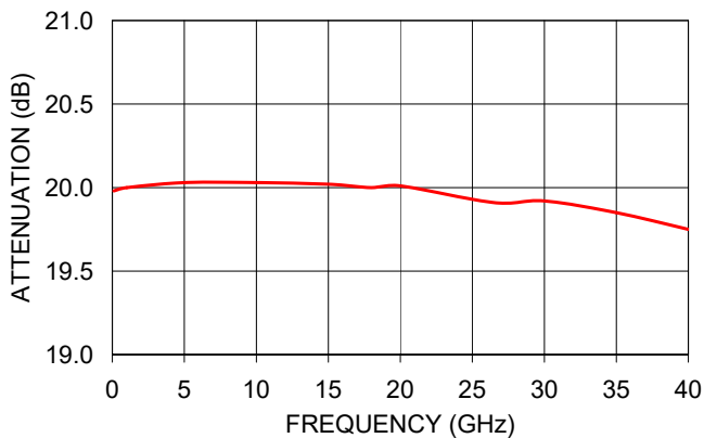
BW-K20-2W44+ ATTENUATION
