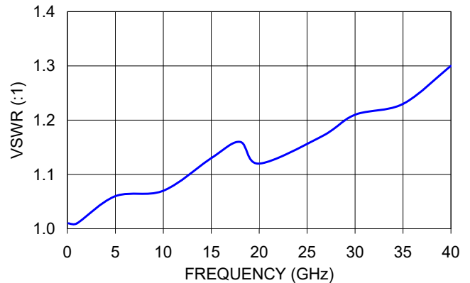
BW-K3-2W44+ VSWR
