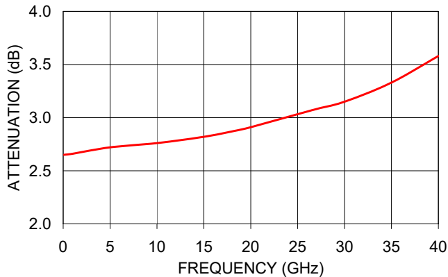
BW-K3-2W44+ ATTENUATION
