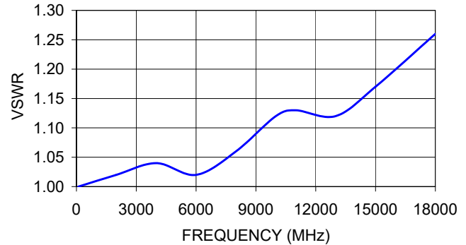
BW-S5W5+ VSWR
