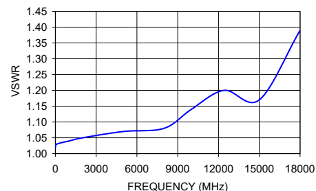
BW-S6W2+ VSWR
