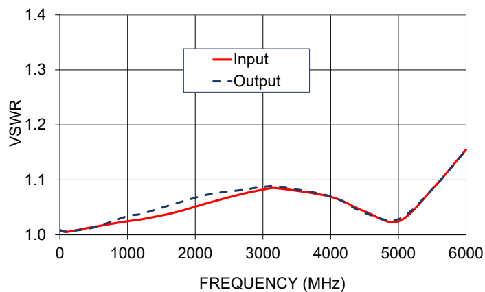
EQY-0-63+ VSWR
