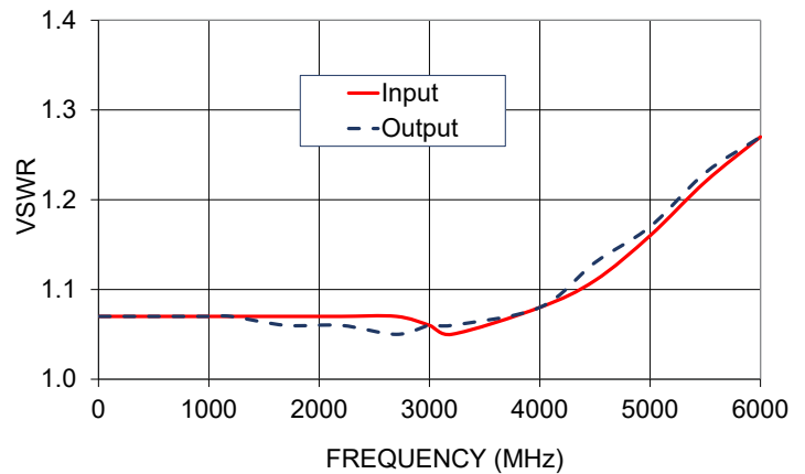
EQY-1-63+ VSWR
