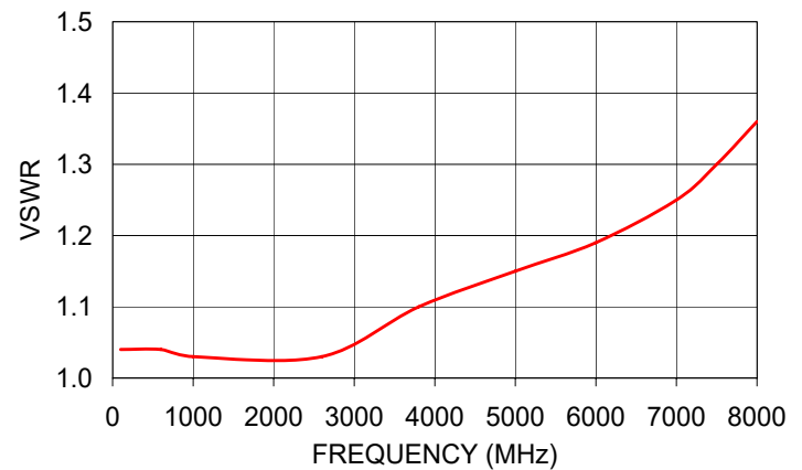
GAT-15+ VSWR
