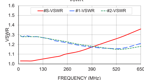
LRPS-2-1W-75+ VSWR
