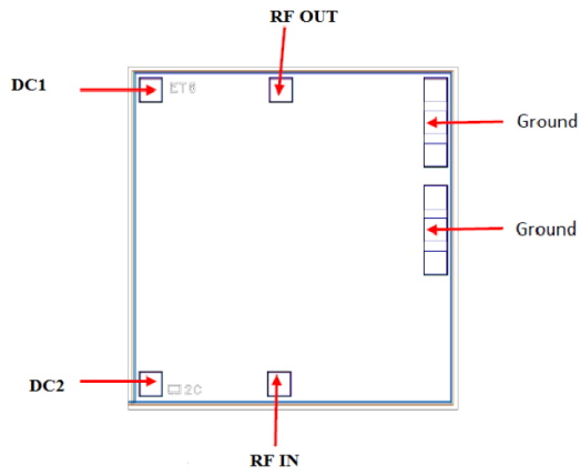
Fig 3. Die Layout
