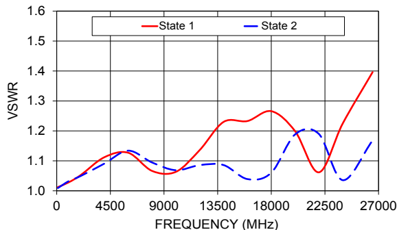
VSWR (J2)
