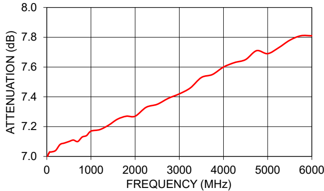
VAT-7W2+ ATTENUATION
