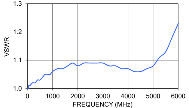
VAT-7W2+ VSWR
