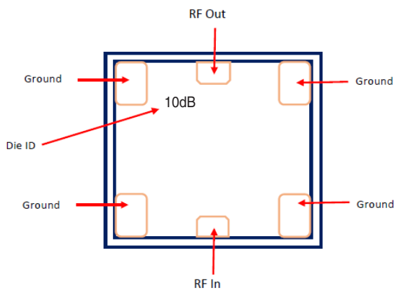
Fig 2. Die Layout Note: Alternate Die ID: ATN3590_10
