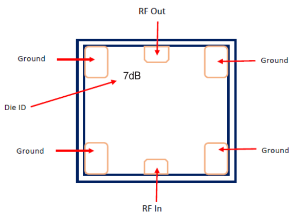
Fig 2. Die Layout
