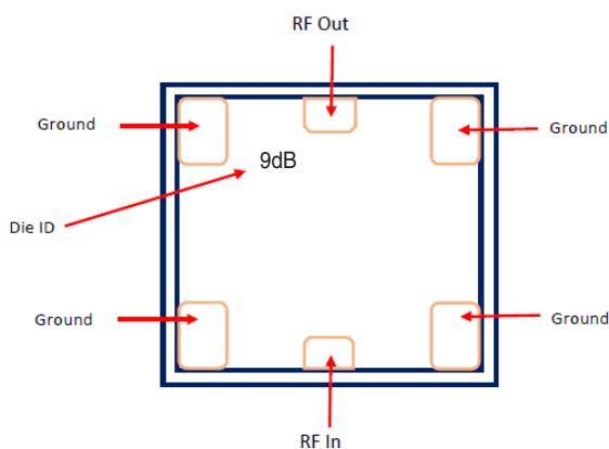
Fig 2. Die Layout Note: Alternate Die ID: ATN3590_09
