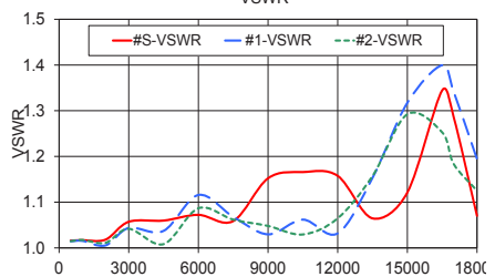
ZFRSC-183-S+ VSWR
