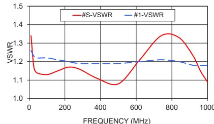
ZFSC-8-43-S+ VSWR
